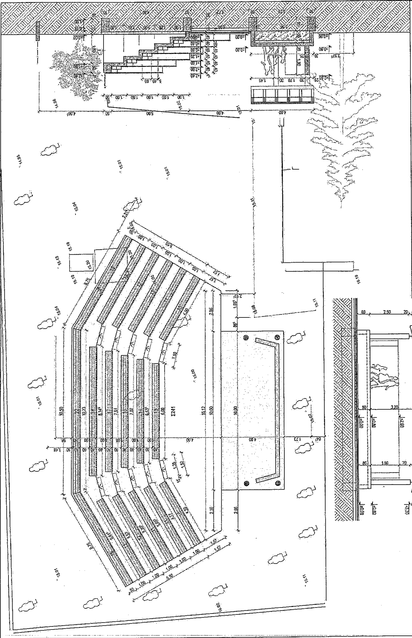
ÁLTALÁNOS ISKOLA SZÍNPAD - VÁZLATTERV - M=1:100
